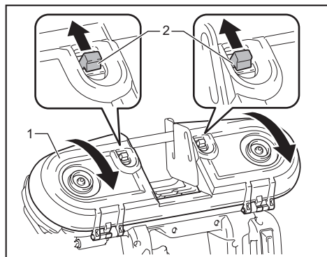
► 1. Capot de meule 2. Crochet
